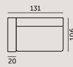
1 SETER XL MED ARM(V) SAP: 294206(H) SAP: 294207(V)
