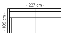
Modul 8 3-seter m/arm V B:227 D:105 H:72 cm SAP: 332646
