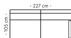
Modul 9 3-seter m/arm H B:227 D:105 H:72 cm SAP: 332647
