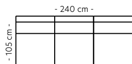
Modul 10 3,5-seter B:240 D:105 H:72 cm SAP: 332632
