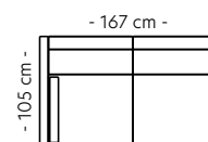
Modul 5 2-seter m/arm V B:167 D:105 H:72 cm SAP: 332643
