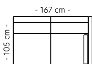
Modul 6 2-seter m/arm H B:167 D:105 H:72 cm SAP: 332644
